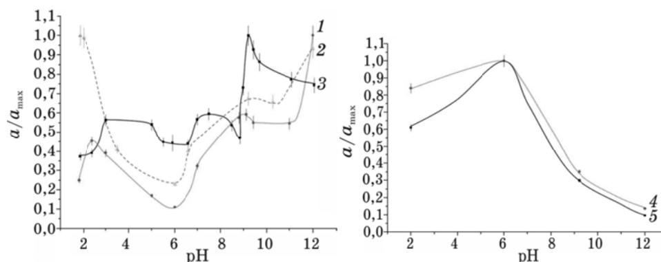
Рис. 1. Залежність питомої сорбції ( a/a_{\max} ) амінокислот від рН для випадку мономолекулярної сорбції: 1 — \alpha -аланін; 2 — \beta -аланін; 3 — гліцин; 4 — триптофан; 5 — L-карбобензоксифенілаланін.
